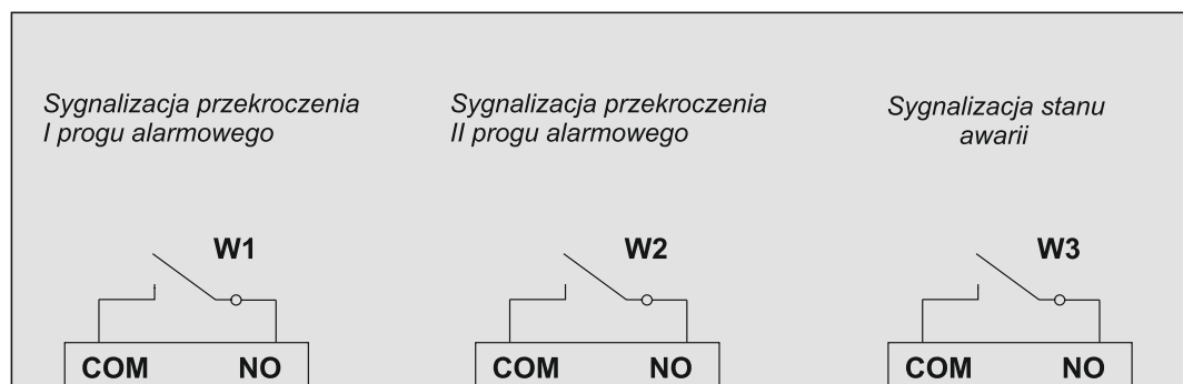
Rys.5. Schemat wyjść stykowych (przełącznikowych) detektora „DUOmaster CO/LPG L”
