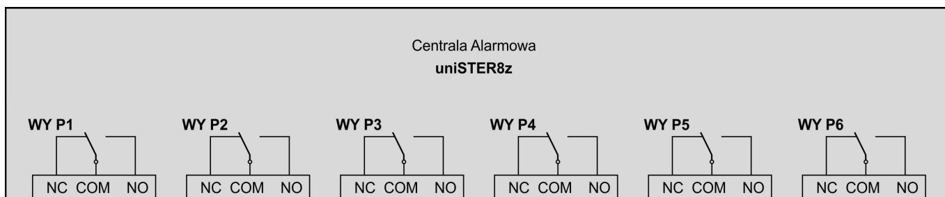
Rys.4. Schemat wyjść stykowych (przekaźnikowych) Centrali Alarmowej uniSTER8z
