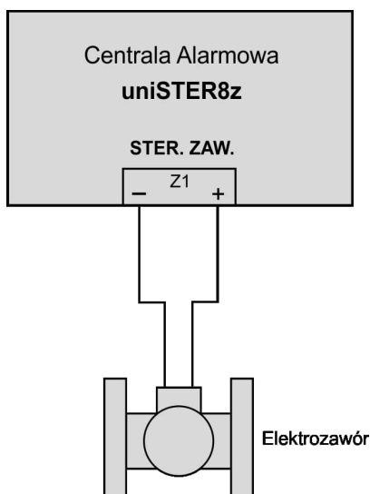
Rys.6. Podłączenie zaworów odcinających (elektrozaworów)
