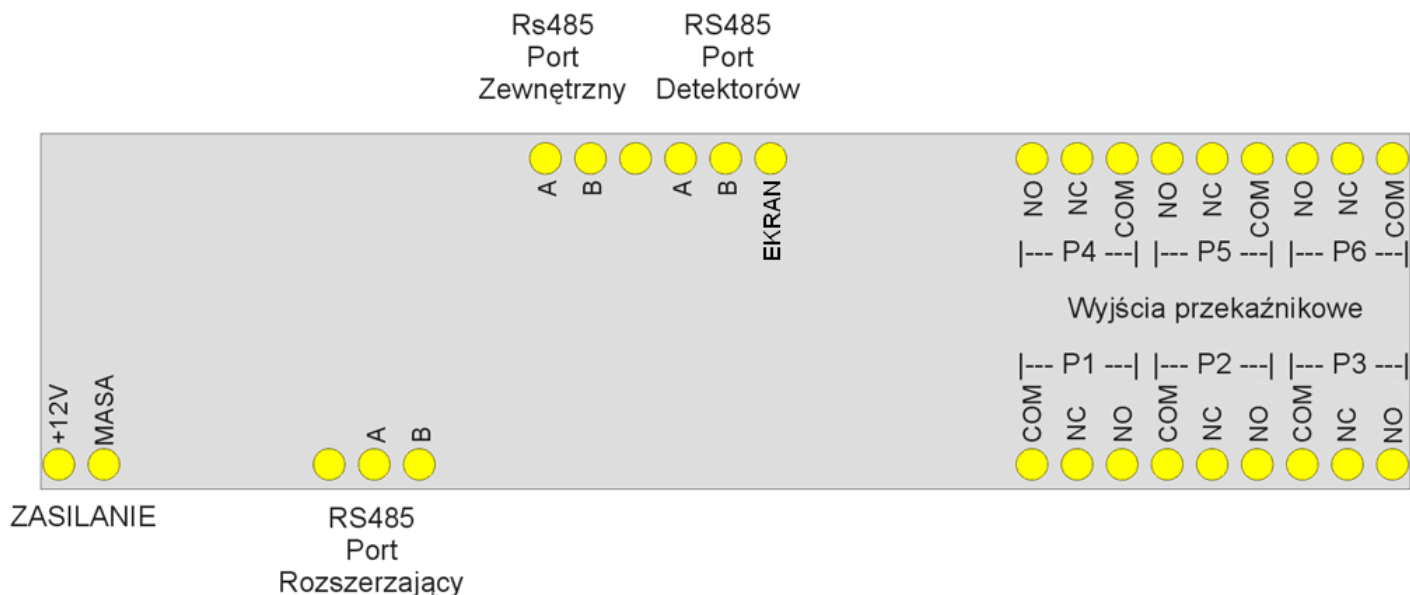
Rys.4. – Opis łączówek modułu DINster.
